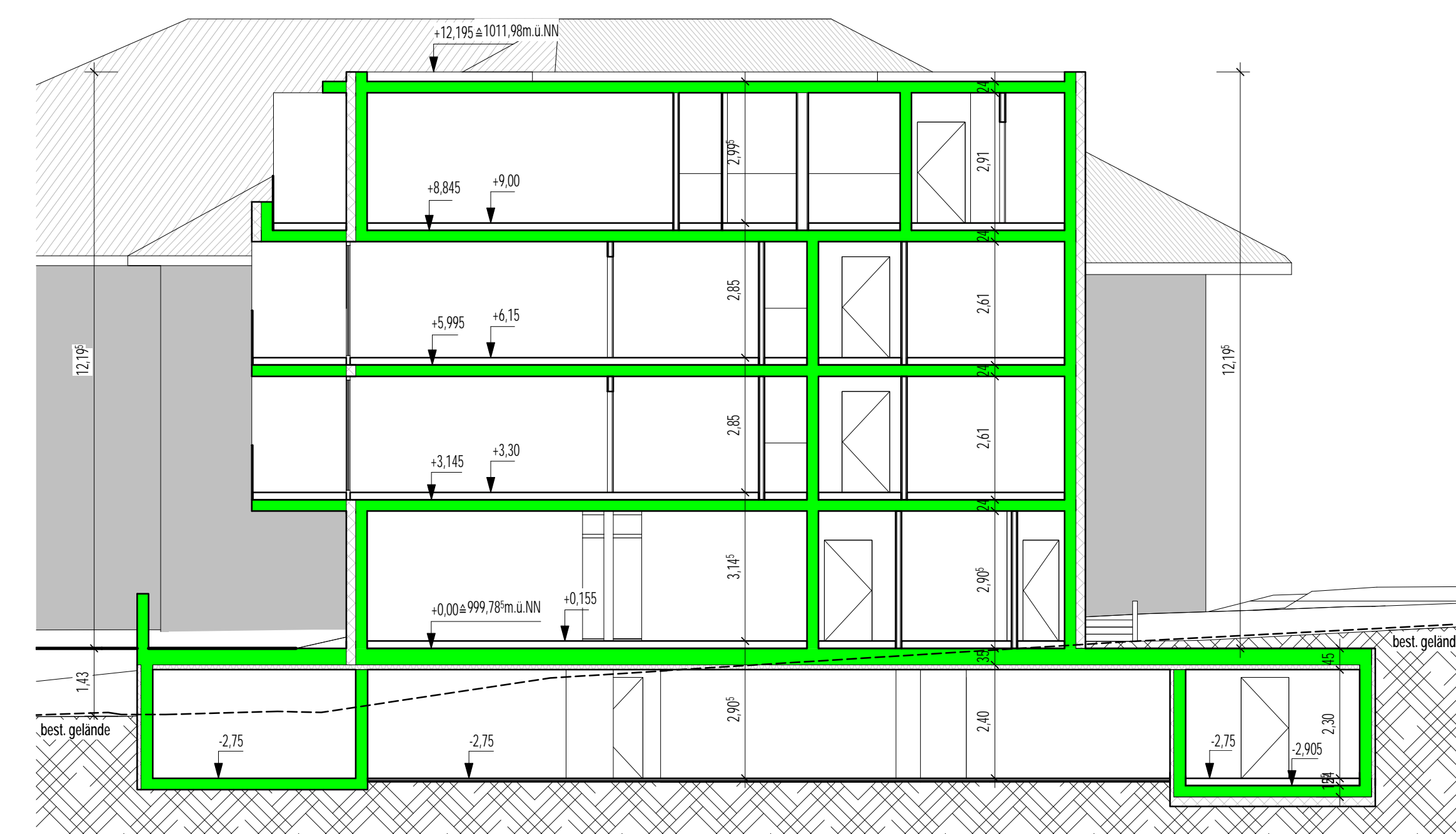
schnitt 1-1
