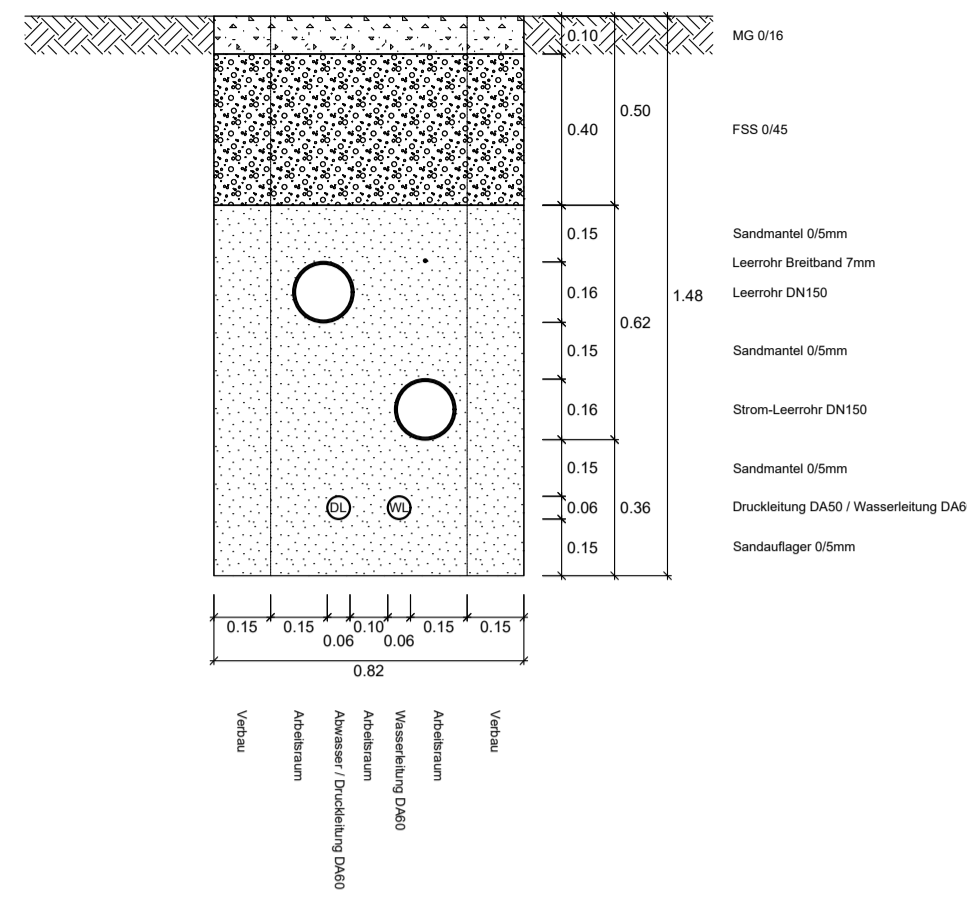
Leitungsgraben RQ ungebunden:
