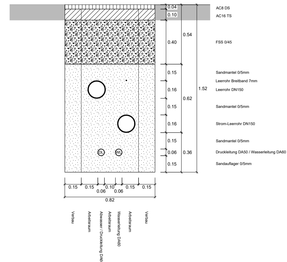
Leitungsgraben RQ gebunden:
